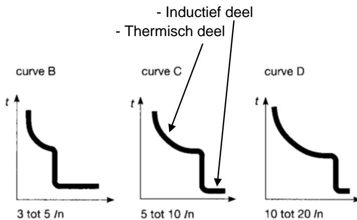
Figuur 8 Uitschakel karakteristiek
