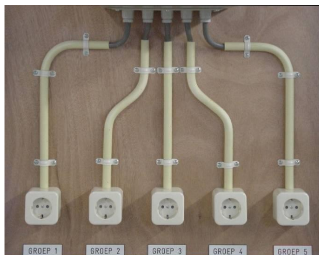
Figuur 16 Wandcontactdozen op de achterkant van de meterkast.
