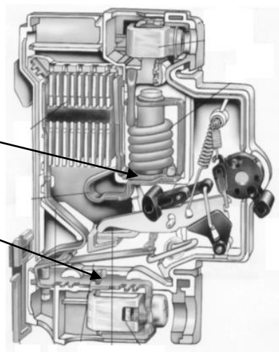
Figuur 7 Binnenwerk installatieautomaat.
