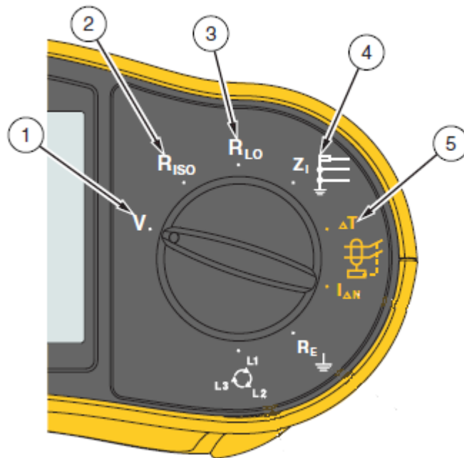
Figuur 17 Meetopdrachten Fluke.
